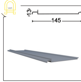
GYTN-1702 Üst Kutu Ön Kapağı Upper Box Cover Profile
