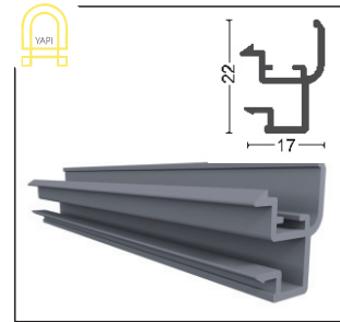
GYTN-1707 Çekme Çıtası Profili Pull Bread Profile
