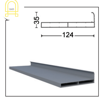
GYTN-1706 Altı Kasa Profili Lower Fram Profile
