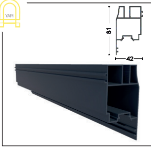
GYTN-1726 Açılır Kanat 8 mm Profile Of Opens 8mm
