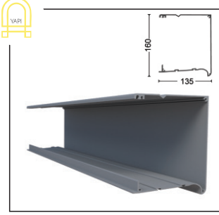
GYTN-1701 Üst Kutu Profili Upper Box Profile
