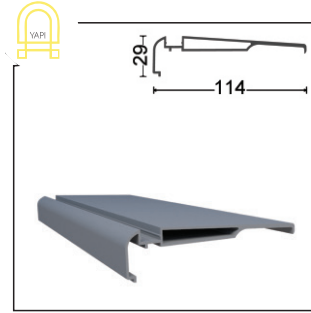
GYTN-1704 Küpeşte Profili Railing Profile
