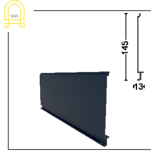
GYTN-1702 Üst Kutu Ön Kapak Upper Box Front Cover
