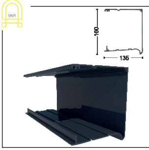
GYTN-1701 Üst Kutu Antrasit Gri Upper Box Anthracite Gray
